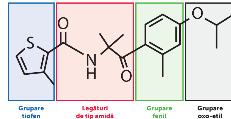
SCHEMA CHIMICĂ
